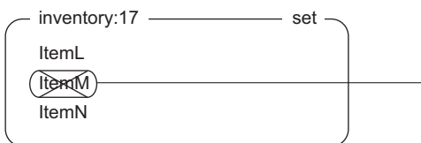
Figure 4.4 list_item(conn, "ItemM", 17, 97)
